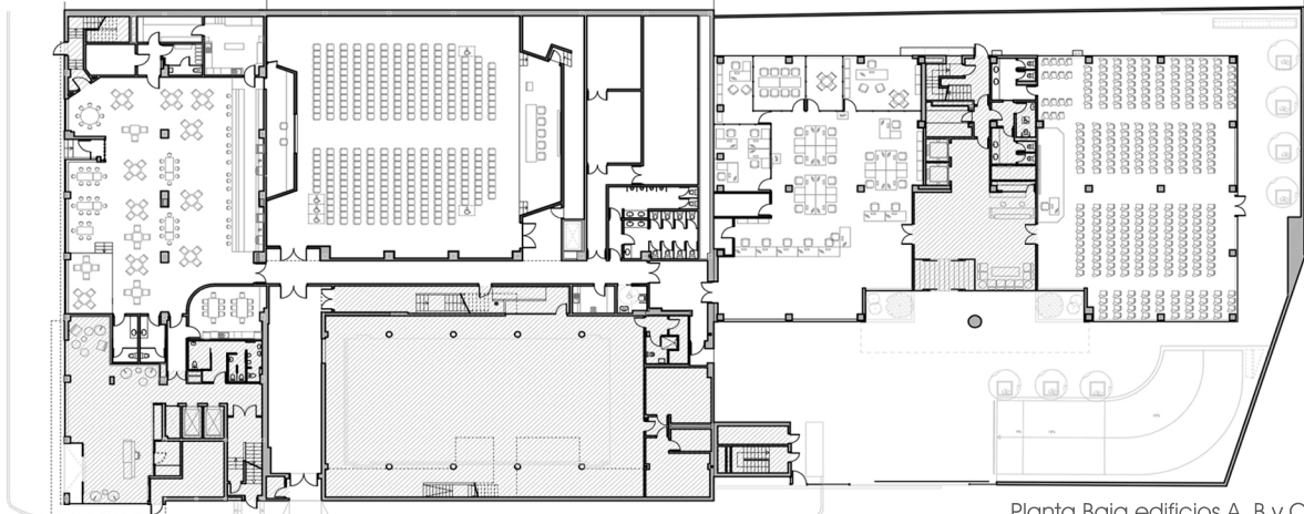
Planta Baja edificios A, B y C
