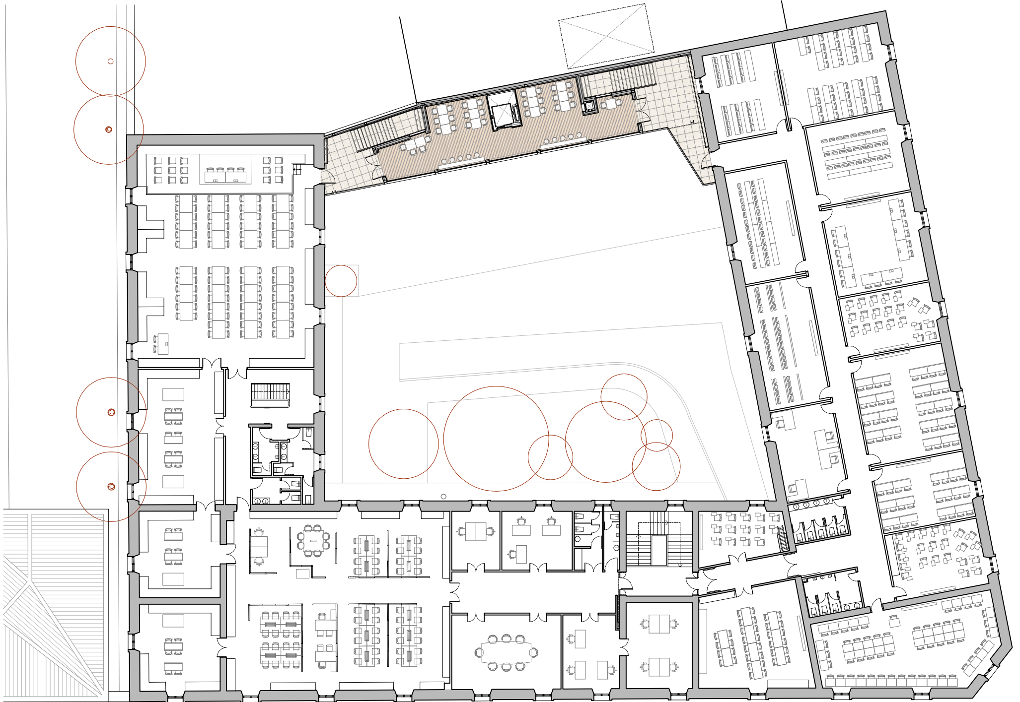
PLANTA PRIMERA
