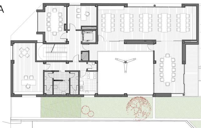
Planta Primera
