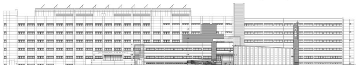
Alzado Noreste
