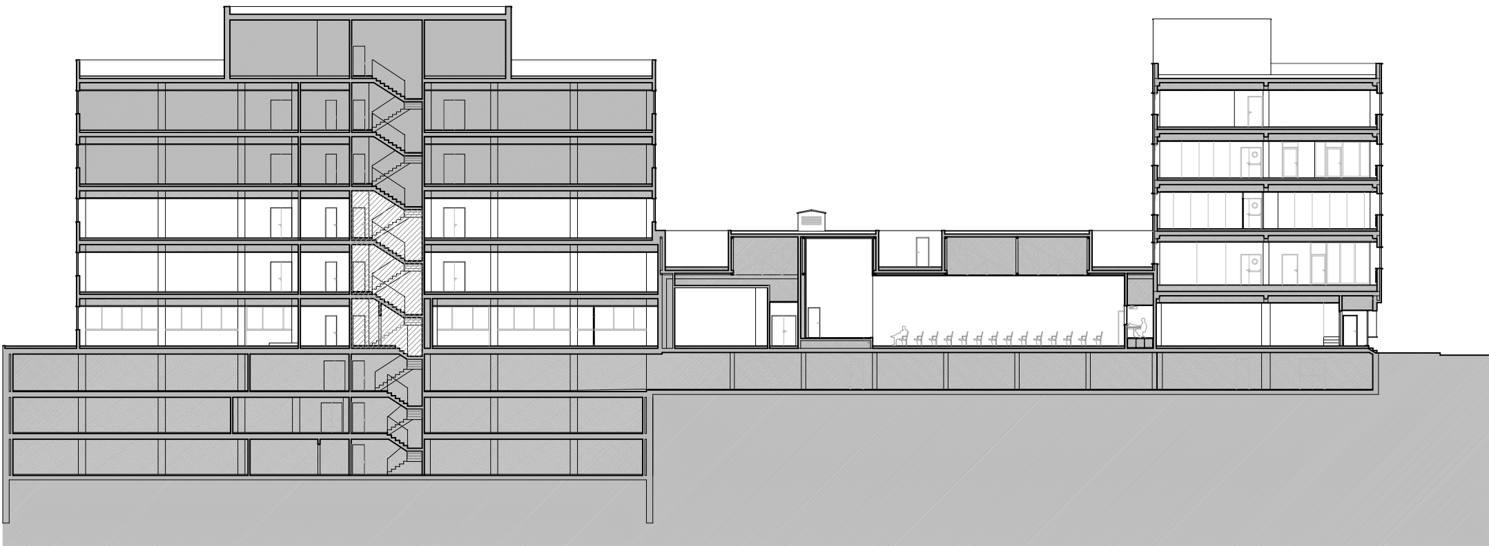
SECCIÓN LONGITUDINAL
